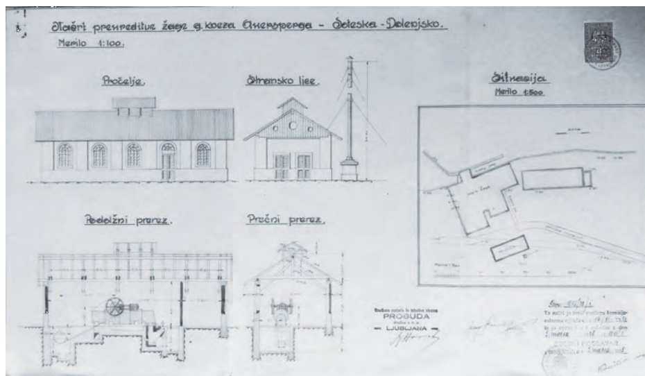
Načrt preureditve žage iz leta 1928
